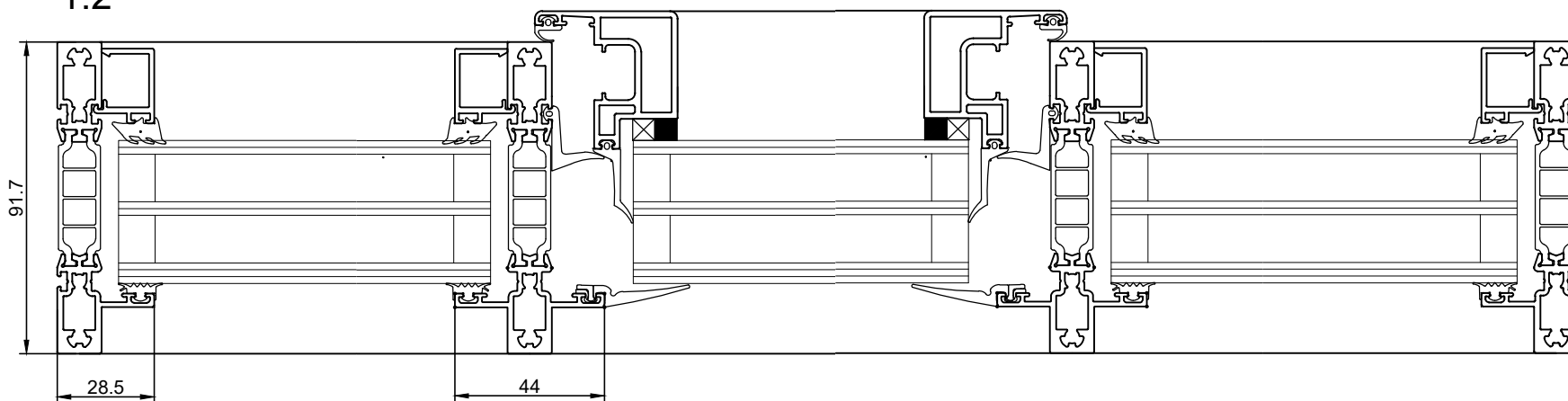
Snit 201 1:2
