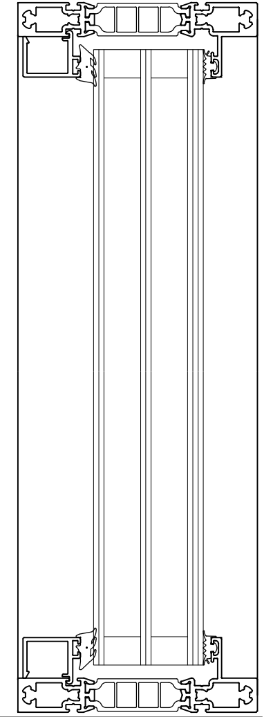
Snit 103 1:2
