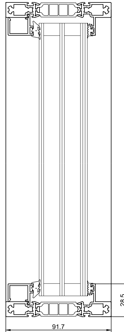
Snit 101 1:2
